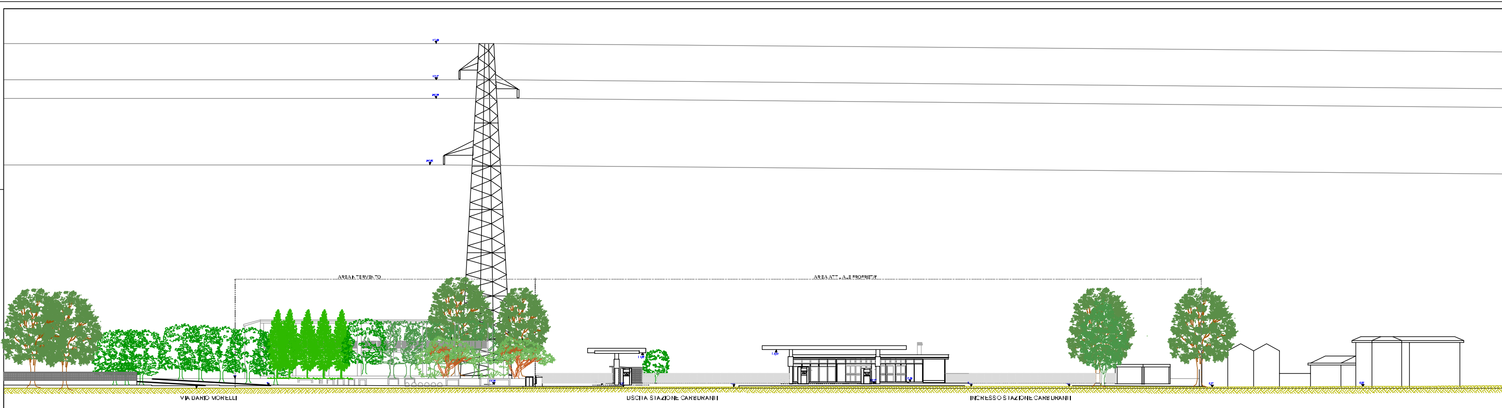
PROSPETTO SU VIA BORGOSATOLLO
