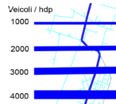
Estratto della Tavola ALall01c – Flussi veicolari – ora di punta del mattino – Stato di fato
