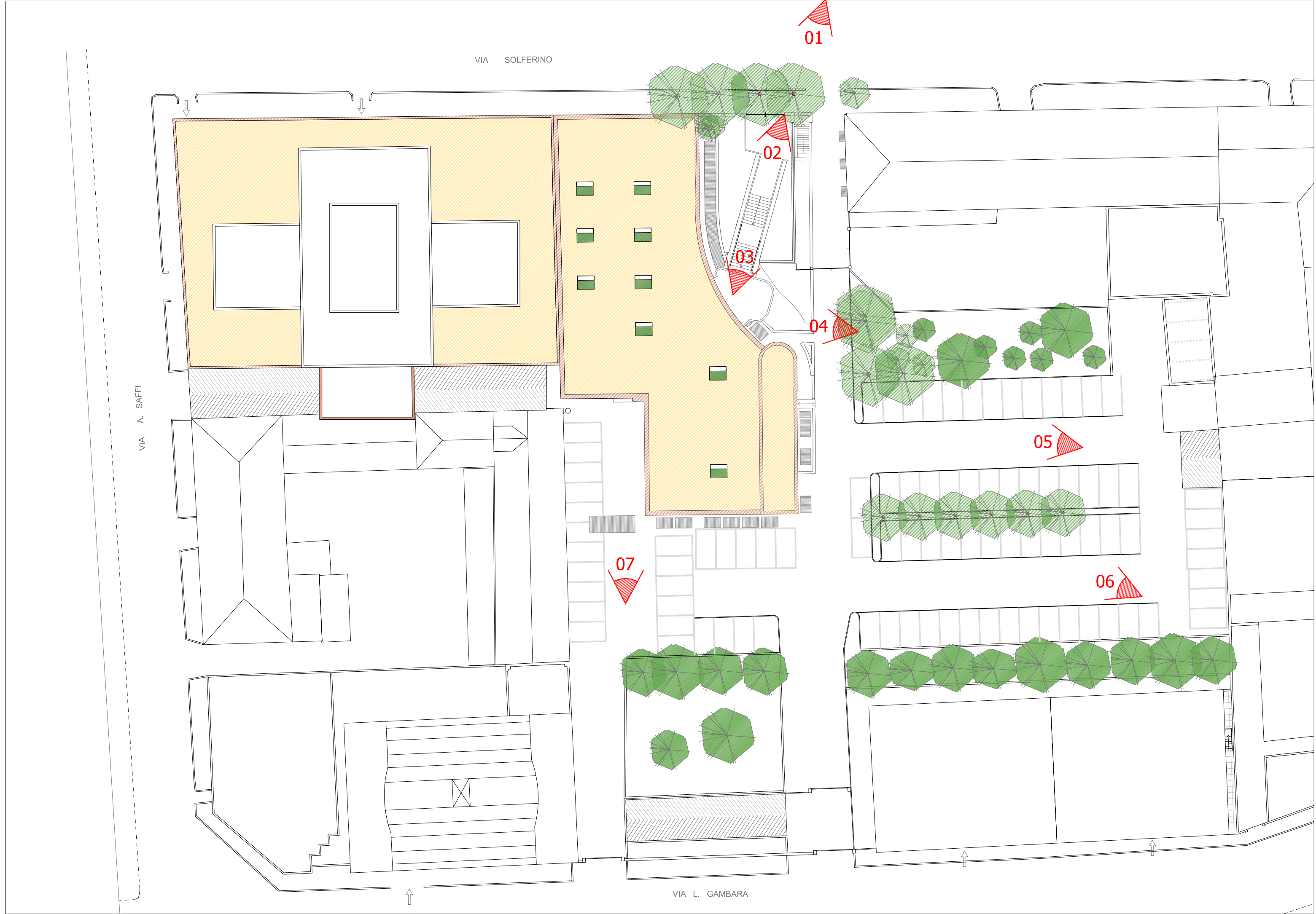
Planimetria scala 1:500
